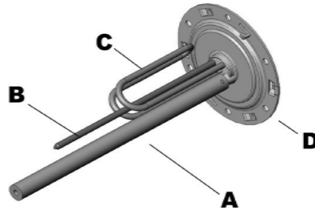
Abbildung 1 - Tauchwiderstand + Magnesiumanode
