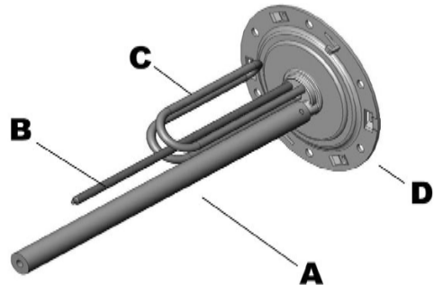
Afbeelding 1 – Dompelweerstand + magnesiumanode
